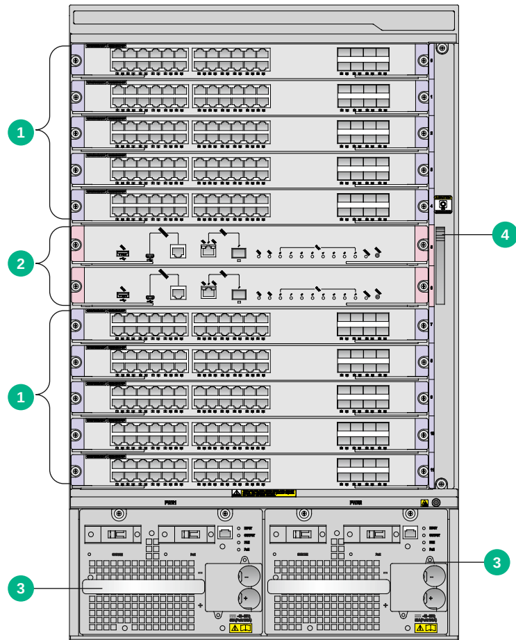
图1-5 S8600X-10-G 前面板示意图
