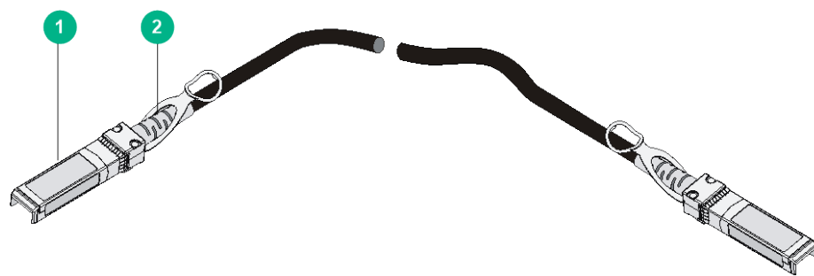
图1-6 SFP+DAC 电缆示意图
