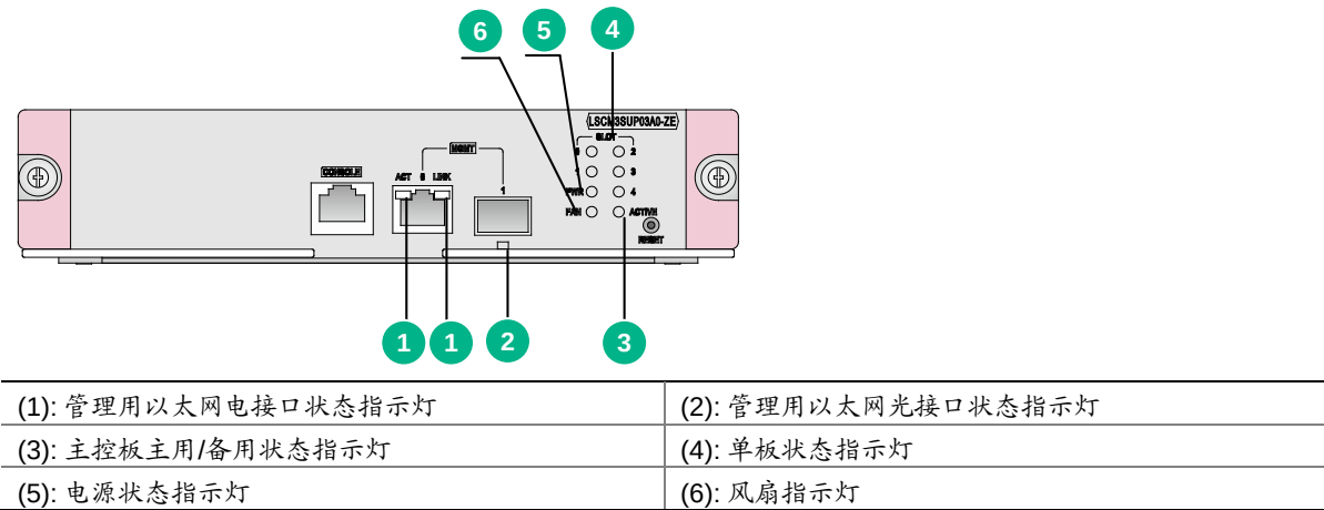
图1-2 LSCM3SUP03A0-ZE 主控板指示灯示意图
