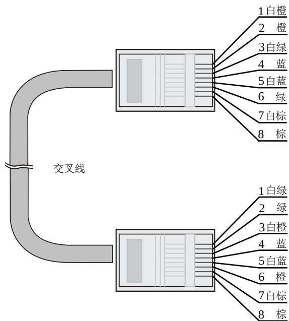
图1-3 交叉线两端线序示意图
