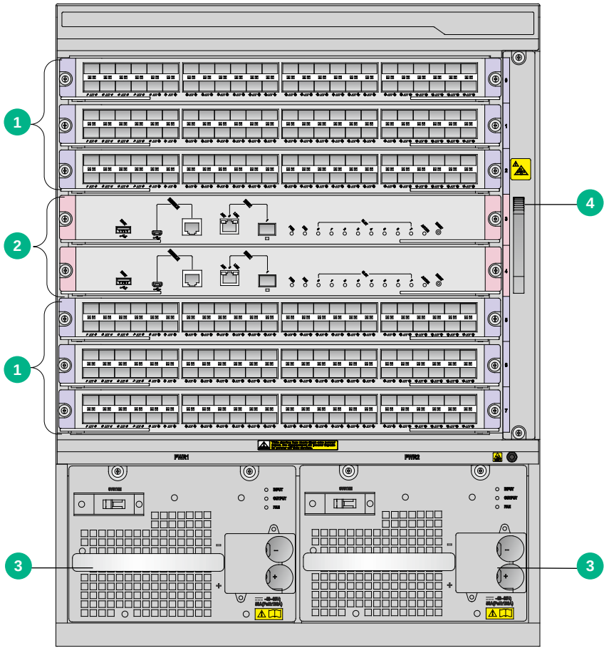
图1-3 S8600X-06-G 前面板示意图
