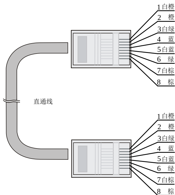
图1-2 直通线两端线序示意图
