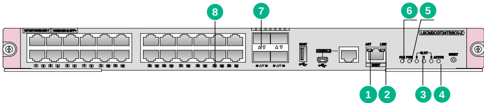
图1-4 LSCM2CGT24TSSC0-Z 主控板指示灯示意图
