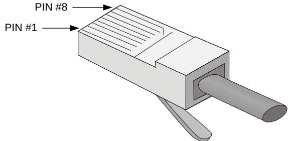
图1-1 RJ-45 连接器引脚序号示意图
