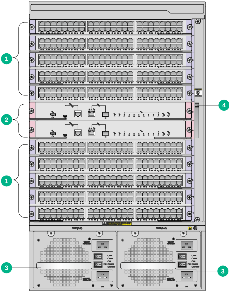
图1-6 S8600X-10-G-PoE 前面板示意图
