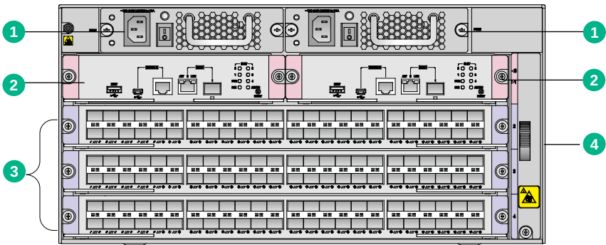
图1-1 S8600X-03-G/S8600X-03-GE 前面板示意图
