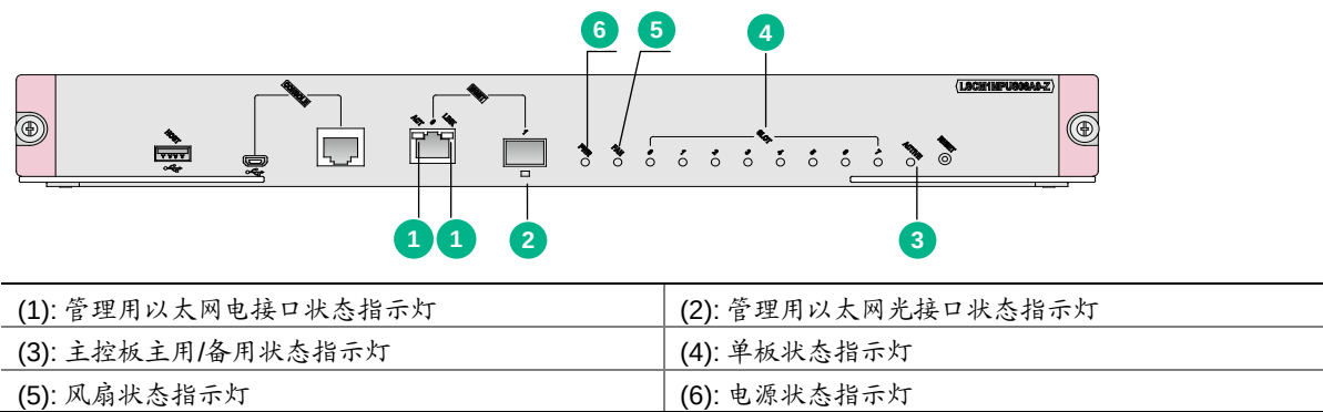
图1-3 LSCM1MPUS06A0-Z 主控板指示灯示意图
