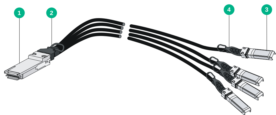
图1-9 QSFP+ to SFP+DAC 电缆示意图
