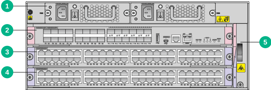
图1-2 S8600X-03M-G 前面板示意图
